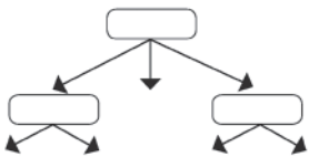
Простая (короткая) гипотеза
