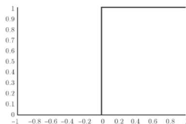
Производная усеченной линейной функции
