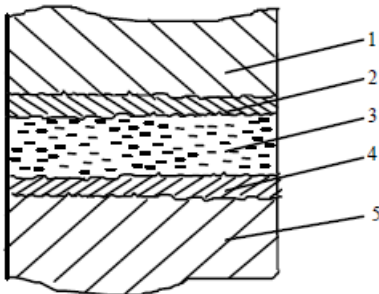
Рис. 2. Структура паяного соединения: 1, 5 – основной металл; 2, 4 – диффузионные зоны; 3 – зона сплавления
