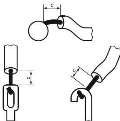
Рис. 22. Размеры освобождения от изоляции
