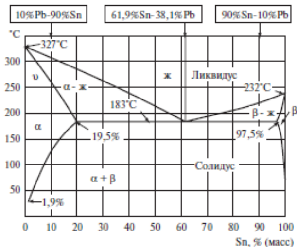
Рис. 4. Диаграмма состояния сплавов олово-свинец
