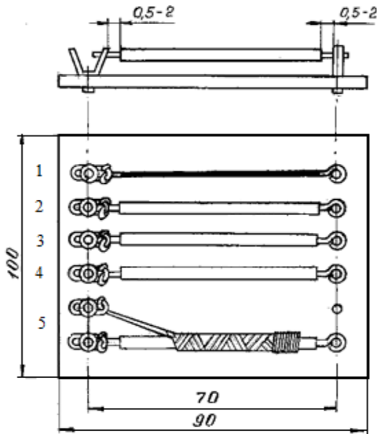
Рис. 3.1. Расположение монтажных проводов на типовой плате: 1 – провод марки ПЭВ; 2 – ПМВ; 3 – МГВ; 4 – МГШ (МЭЦДЛ); 5 – МГШВЛЭ
