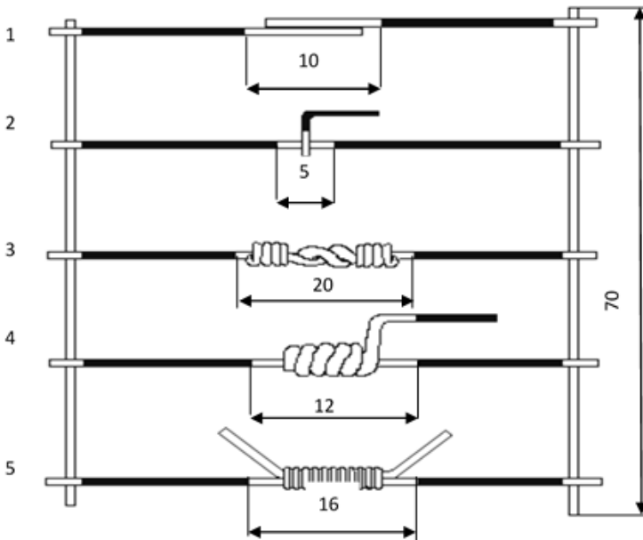
Рис. 2.1. Типы монтажных соединений жил проводов: 1 – соединение внахлест двух проводников; 2 – колечком (отвод от основного провода); 3 – скрутки двух проводов; 4 – навивкой (отвод от основного провода); 5 – бандажированием
