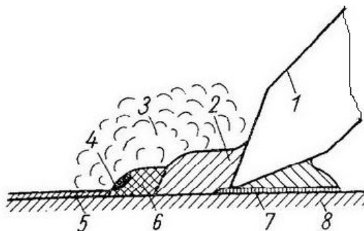
Рис. 7. Процесс горячего лужения с помощью паяльника:
