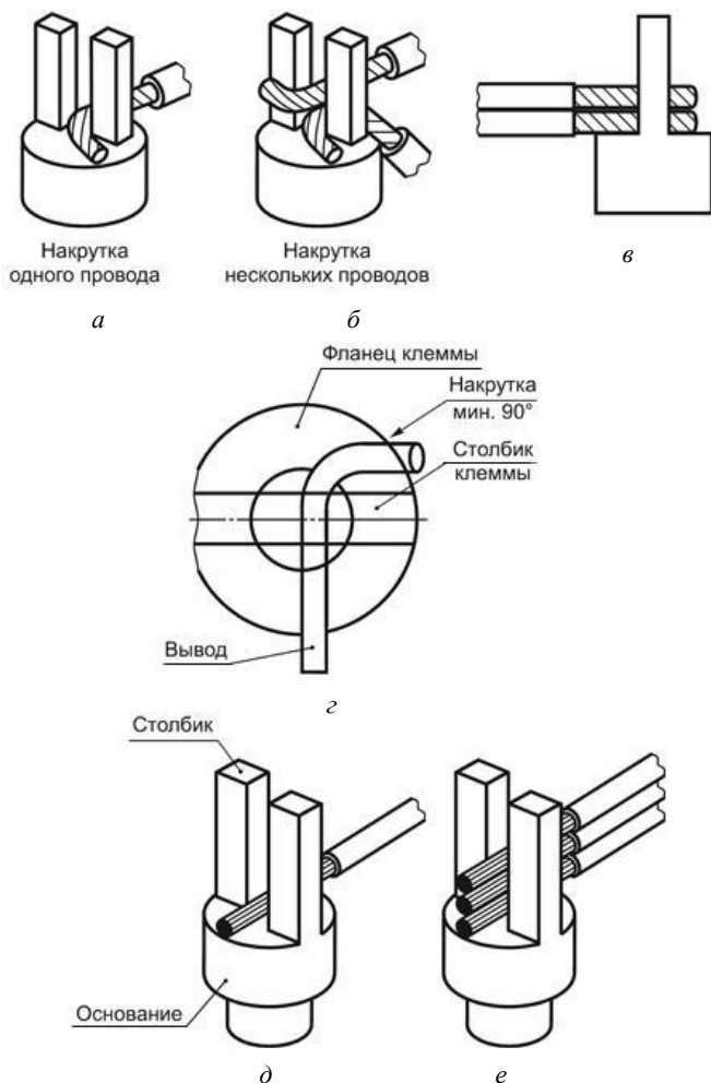
Рис. 20. Монтаж в разрезной контакт
