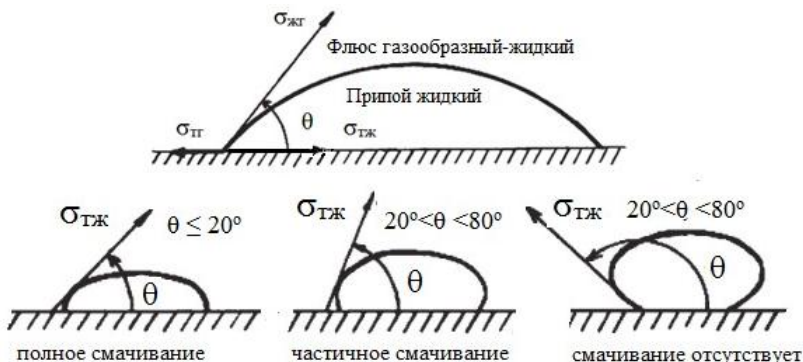
Рис. 1. Схема равновесия сил поверхностного натяжения
