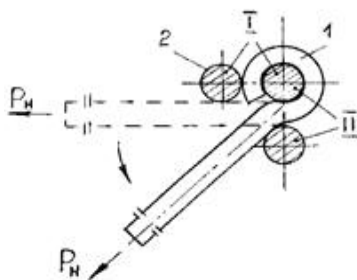
Рис. 2.2. Формовки колечка с применением круглогубцев
