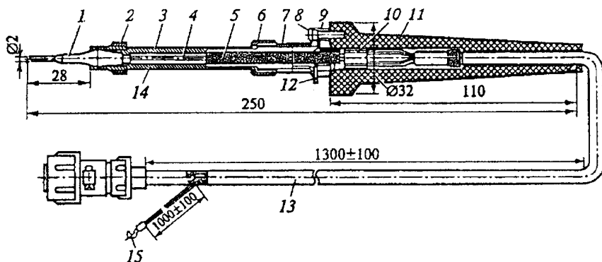
Рис. 8. Конструкция электропаяльника с заземлением: 1 – наконечник; 2, 6 – гайки; 3 – трубка; 4 – термopара; 5 – керамическая трубка; 7 – основание; 8 – винт; 9 – втулка; 10 – термостойкие изоляционные трубки; 11 – ручка; 12 – держатель (пластина); 13 – жгут из проводов питания, термopары и заземления; 14 – нагревательный элемент; 15 – провод для заземления.
