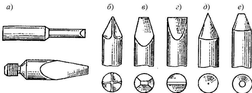
Рис. 9. Типы паяльных наконечников (а) и формы заточки их рабочей части: б – пирамидка; в – четырехгранный клин; г – клин; д – конус; е – срезанный конус
