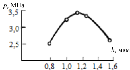
Рис. 3. Изменение прочности паяных соединений в зависимости от ширины диффузионной зоны
