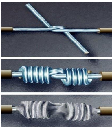
Рис. 2.3. Соединение проводов скруткой
