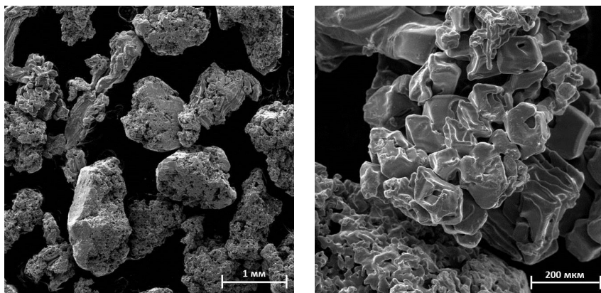
Рис. 6.2. Форма порошкового титана ТПП-4 (ТУ 14-22-57-98)
