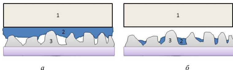
Рис. 3.6. Варианты воздействия при соединении поверхностей вязким клеем (а) и жидким клеем (б): 1 – компактный склеиваемый материал; 2 – клей; 3 – пористый склеиваемый материал
