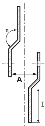
Рис. 4.2. Принципиальная схема приспособления для проведения испытаний на условный сдвиг
