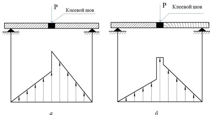
Рис. 3.4. Схема эпюры прогиба при деформации пластины, склеенной вязким клеем:
