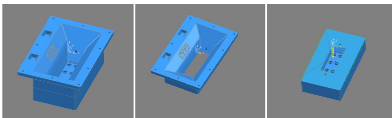
Рис. 5.22. Изображение модели отливки «Корпус»
