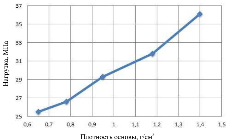
Рис. 3.7. Прочность на растяжение пластических масс различной плотности, склеенных клеем DP 8005 (3M)
