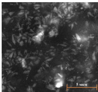
Рис. 6.10. Структура акрилового адгезива типа DP 8805NS
