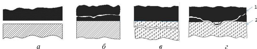
Рис. 4.1. Виды разрушений адгезионных соединений:
