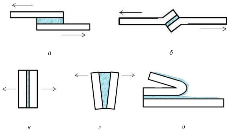
Рис. 3.2. Основные типы нагружения клевого соединения: a, б – сдвиг; в – равномерный отрыв; г – внецентровой отрыв; д – отдир
