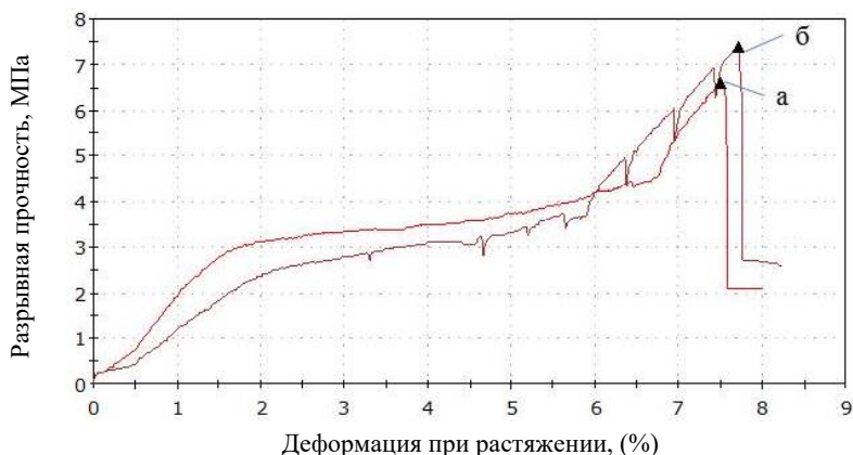
Рис. 6.17. Диаграмма растяжения образцов МПТМ, прошедшие испытания на разрыв, после искусственного старения адгезионного клевого соединения (клей DP 8805NS) в условиях масляной среды: а – группа образцов d_{\text{фракций}} = 0,40\text{--}0,63 мм без дополнительной защиты клевого шва; б – группа образцов d_{\text{фракций}} = 0,40\text{--}0,63 мм с дополнительной защитой клевого шва при помощи лакокрасочных изделий
