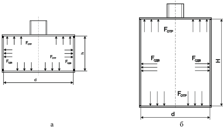
Рис. 4.6. Модели для проведения гидро- или пневматических испытаний: a – модель для проведения испытаний на условный отрыв; б – модель для проведения испытаний на условный сдвиг
