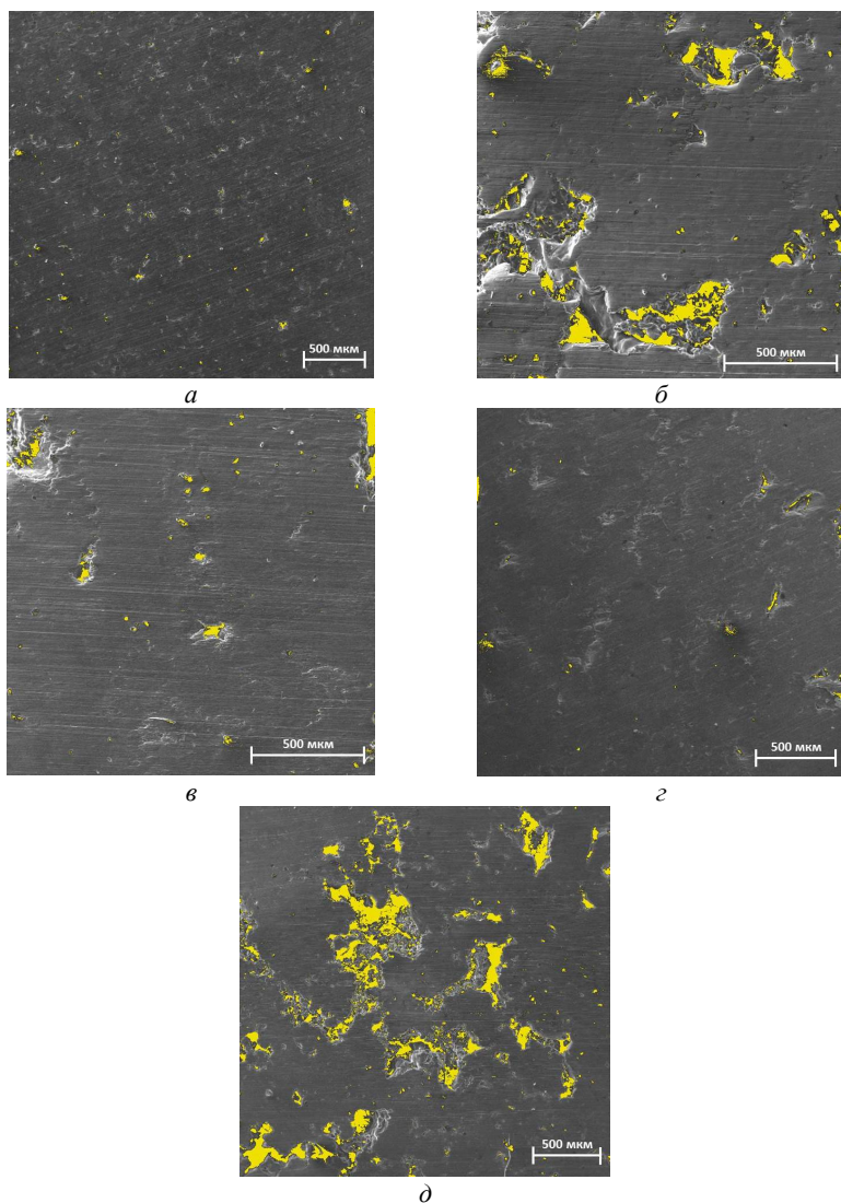
Рис. 6.4. Макроструктура поверхностного слоя исходных титановых таблеток с поверхностной пористостью: a – 20–25 %; б – 30–35 %; в – 28–32 %; г – 28–32 %; д – 40 %
