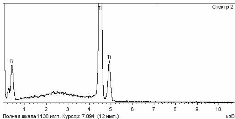
Рис. 6.3. Спектральные составляющие порошка титана марки ТПП4 (ТУ 1422–57–98)
