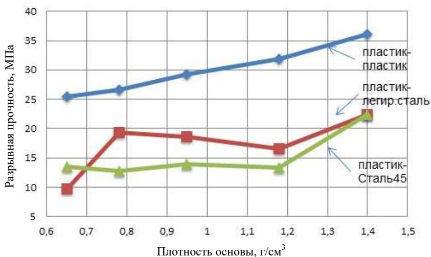
Рис. 5.11. Образцы, склеенные клеем на акриловой основе
