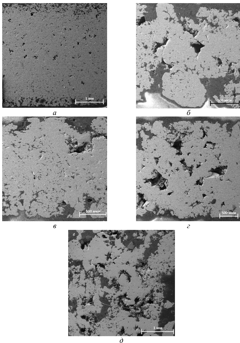
Рис. 6.6. Макроструктура образцов, на основе пористого тела (вверху) и цельного металла (внизу), склеенные акриловым клеем марки DP 8805NS: a – 20–25 %; б – 30–35 %; в – 28–32 %; г – 28–32 %; д – 40 %
