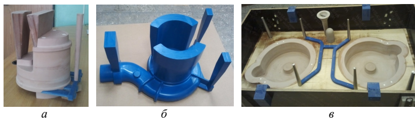
Рис. 5.3. Примеры исполнения модельной оснастки:
