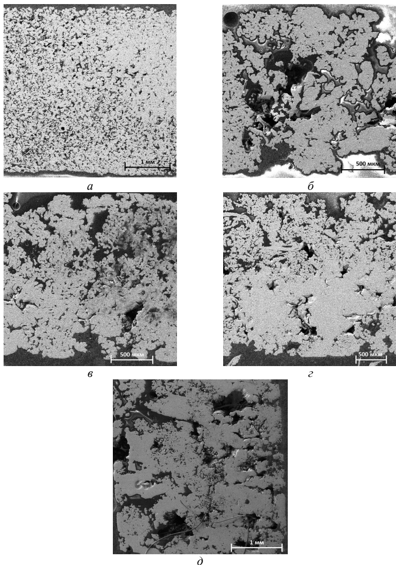
Рис. 6.5. Макроструктура образцов, на основе пористого тела (вверху) и цельного металла (внизу), склеенные эпоксидным клеем марки DP 270: a – 20–25 %; б – 30–35 %; в – 28–32 %; г – 28–32 %; д – 40 %
