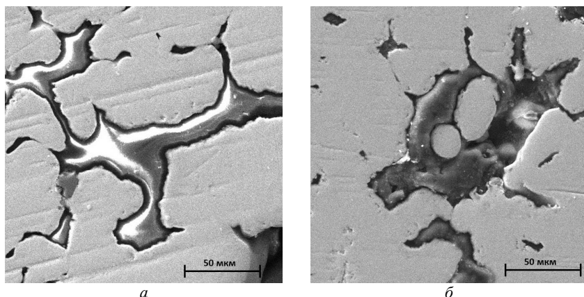
Рис. 6.8. Клеевые мениски в порах титановой губки а – эпоксидная основа, б – акриловая основа
