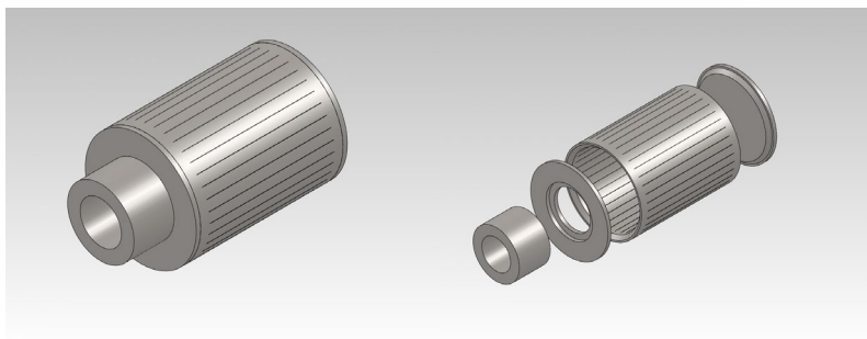
Рис. 4.7. Сборочная схема щелевого фильтра
