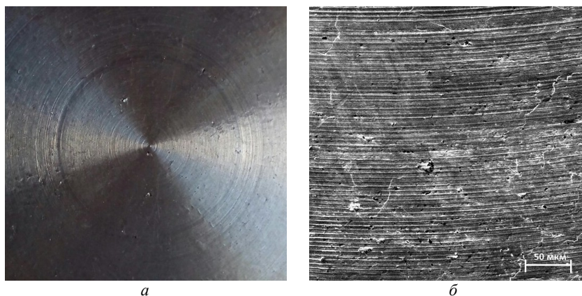
Рис. 6.12. Поверхность образца пористого титана с размером фракций порошка 0,4–0,63 мм, подвергнутая механической обработке: a – общий вид поверхности образца; б – образец при увеличении \times 65
