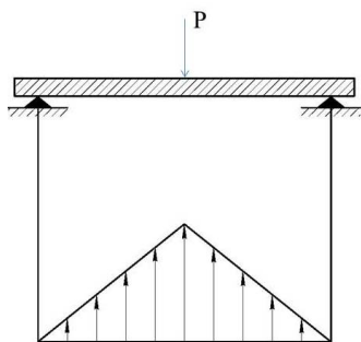
Рис. 3.3. Схема эпюры прогиба при деформации однородной пластины
