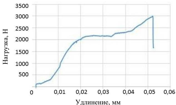
Рис. 6.16. Диаграмма растяжения образцов МПТМ, прошедшие испытания на разрыв, после искусственного старения адгезионного клеевого соединения (акриловый клей DP 8805NS) в условиях водной среды с использованием промежуточного внутреннего клеевого слоя
