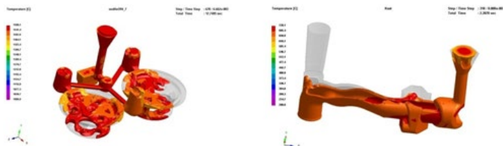
Рис. 5.18. Имитационное моделирование процесса заливки и кристаллизации отливки
