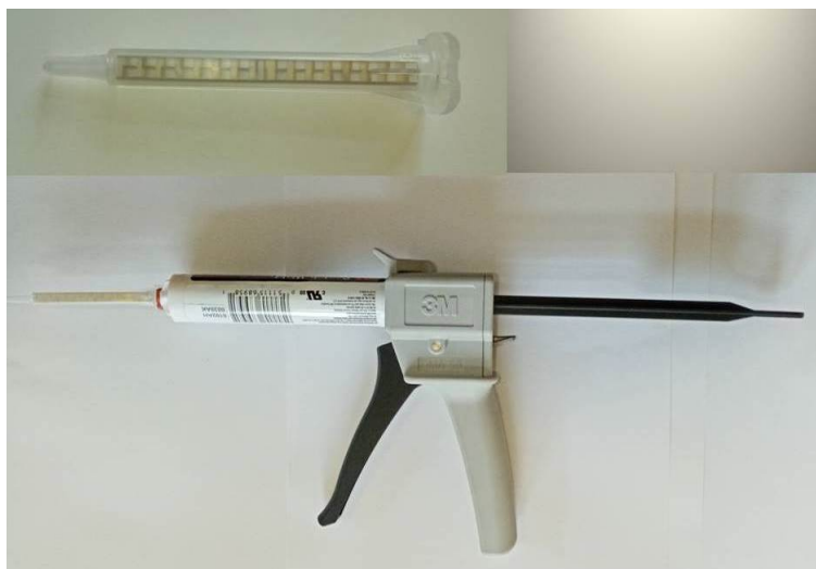
Рис. 3.8. Ручной аппликатор для двухкомпонентных клеев с насадкой
