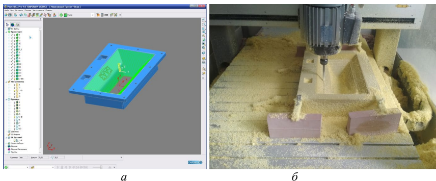
Рис. 5.24. Чистовая обработка заготовки: а – вид диалогового окна PowerMill; б – обрабатываемая заготовка на рабочем столе
