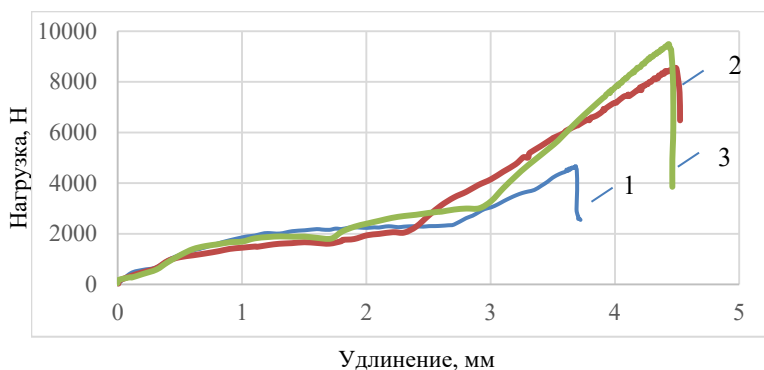
Рис. 6.11. Диаграмма растяжения группы образцов МПТМ, соединенных клеем DP 8805NS:
