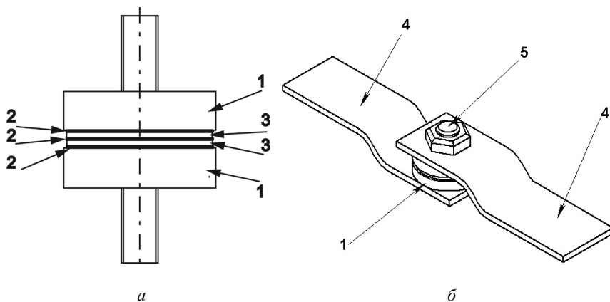
Рис. 4.3. Образец и приспособление для проведения механических испытаний многомерного композиционного соединения: а – образец в собранном состоянии; б – образец, закрепленный в приспособление; 1 – подложки, которые также являются опорными (несущими) составляющими образца; 2 – соединяющий слой (испытываемое связующее); 3 – набор изучаемых композиционных элементов; 4 – приспособление из высокопрочных материалов; 5 – гайка для крепления образца к оснастке
