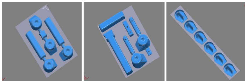
Рис. 5.20. Компоновка элементов литниковой системы
