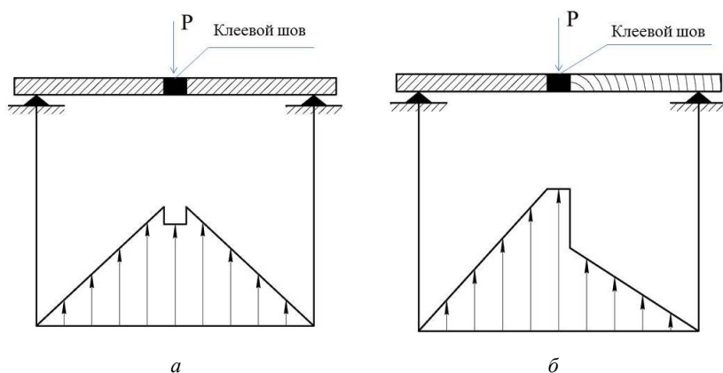
Рис. 3.5. Схема эпюры прогиба при деформации пластины, склеенной высокопрочным клеем:
