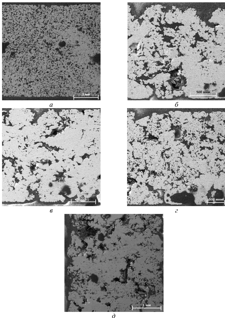
Рис. 6.7. Макроструктура образцов, на основе пористого тела (вверху) и цельного металла (внизу), склеенные эпоксидным универсальным клеем марки ЭДП: a – пористость 20–25 %; б – 30–35 %; в – 28–32 %; г – 28–32 %; д – 40 %
