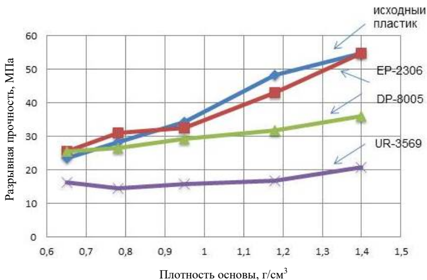
Рис. 5.5. Усредненная прочность на растяжение соединений пластик/пластик, склеенных различными видами клея
