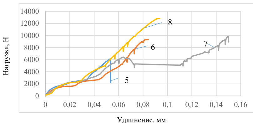
Рис. 6.13. Диаграмма растяжения группы образцов МПТМ, соединенных клеем DP 8805NS:
