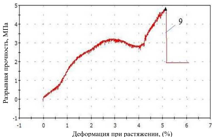
Рис. 6.14. Диаграмма растяжения группы образцов МПТМ, соединенных клеем DP 8805NS с использованием промежуточного внутреннего клеевого слоя
