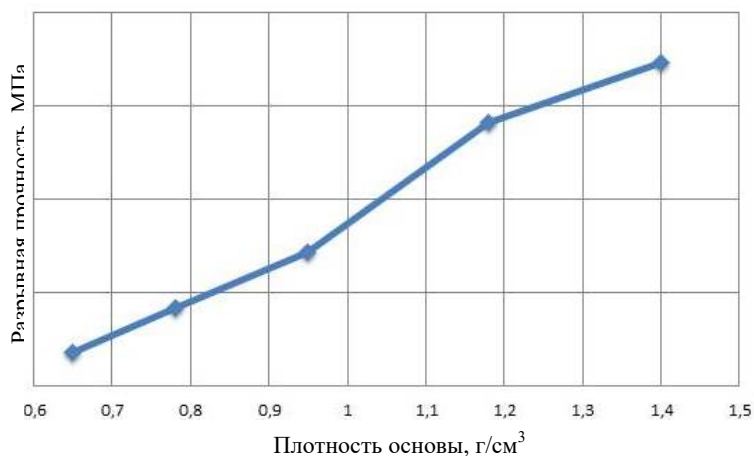
Рис. 5.4. Усредненная прочность некоторых видов исходного пластика при испытаниях на растяжение
