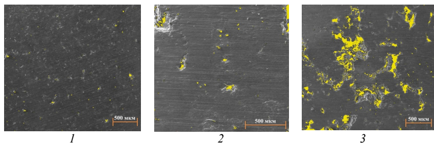
Рис. 6.9. Макроструктура исходных титановых образцов: 1 – образец d_{\text{фракций}} = 0,10\text{--}0,16 мм; 2 – образец d_{\text{фракций}} = 0,4\text{--}0,63 мм; 3 – образец d_{\text{фракций}} = 0,63\text{--}1,0 мм
