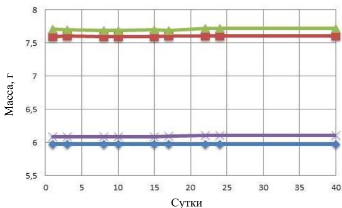
Рис. 6.15. Изменение массы образцов при выдержке в водной среде
