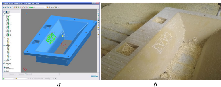
Рис. 5.25. Доработка заготовки: а – вид диалогового окна PowerMill; б – фрагмент обрабатываемой заготовки на рабочем столе
