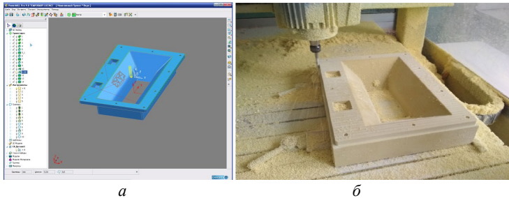
Рис. 5.26. Обработка плоскостей заготовки: а – вид диалогового окна PowerMill; б – обрабатываемая заготовка на рабочем столе
