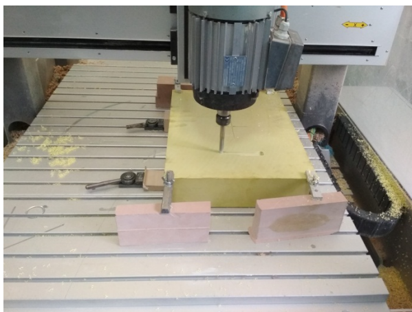
Рис. 5.21. Рабочий стол станка с установленной заготовкой
