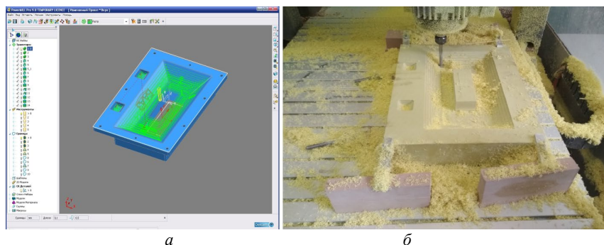
Рис. 5.23. Черновая обработка заготовки: а – вид диалогового окна PowerMill; б – обрабатываемая заготовка на рабочем столе
