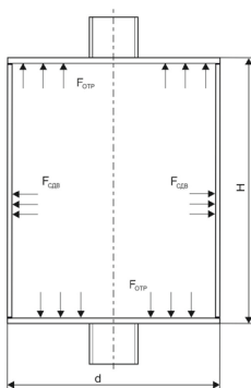
Рис. 4.12. Схема двухштуцерной модели для проведения гидравлических или пневматических испытаний
