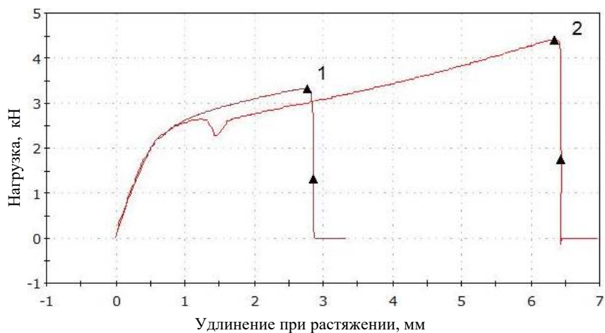
Рис. 4.5. Диаграмма растяжения образцов склеенных клеем DP 8805NS: 1 – образец, на подложку которого были нанесены бороздки; 2 – образец с гладкой поверхностью подложки
